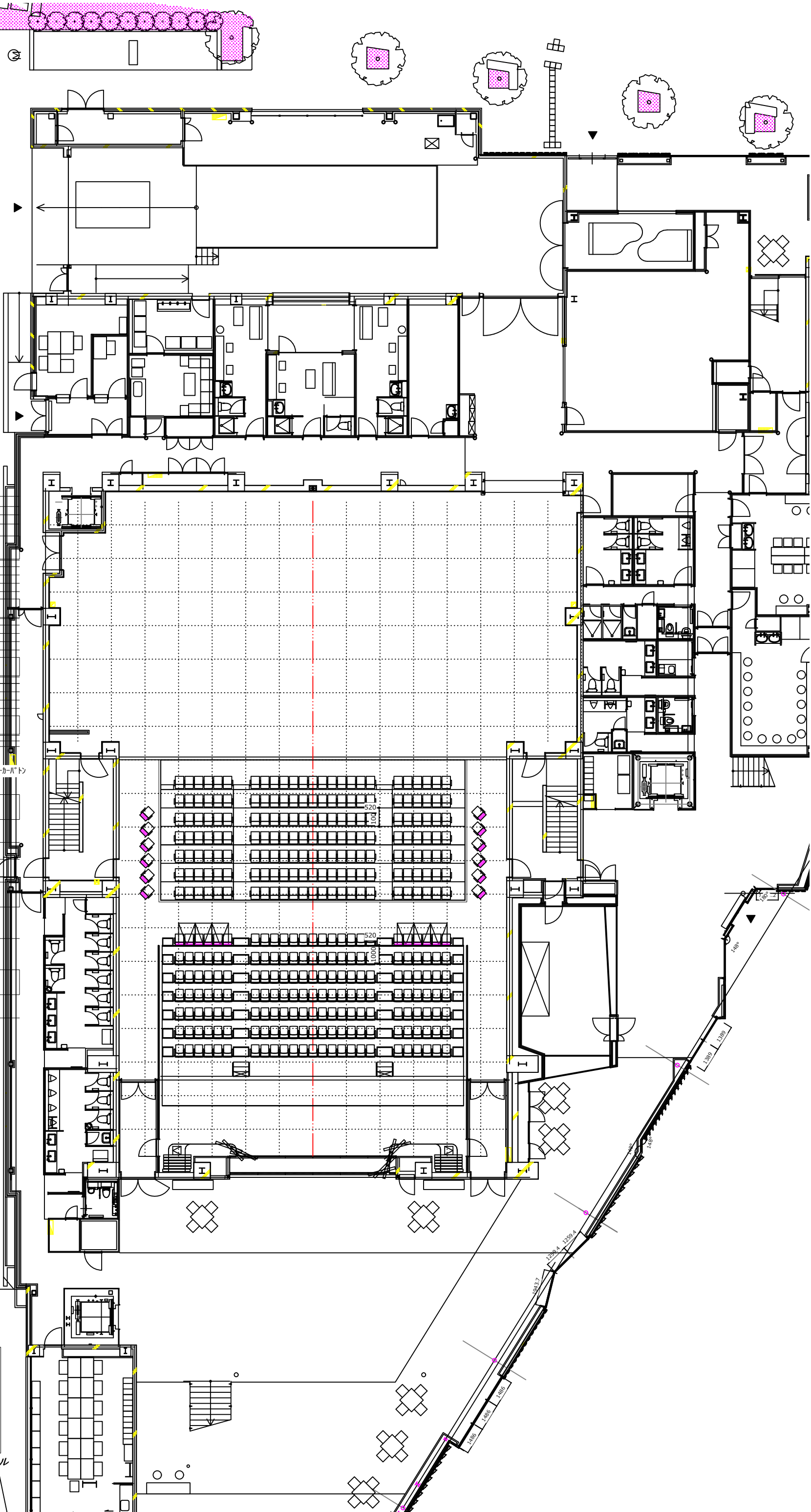
舞台平面図 中ホール S=1:200 AUBADE HALL 富山市芸術文化ホール
